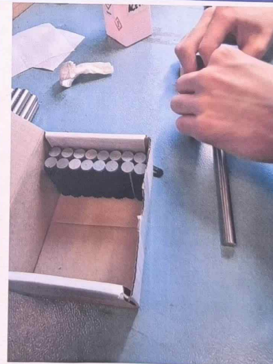
Magneten werden mit Aceton gesäubert und dann mit Klettverschlüssen beklebt.
